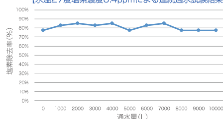
【水温27度塩素濃度0.4ppmによる連続通水試験結果】
